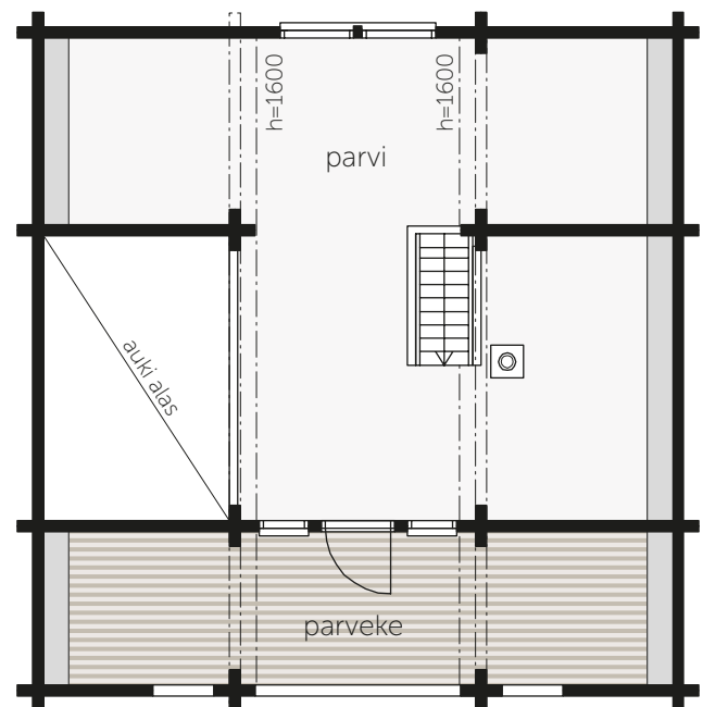
Hongisto A3 parven pohjakuva. Muiden variaatioiden parvien pohjakuvat ja yksikerrosversiot löydät www.kontio.fi
