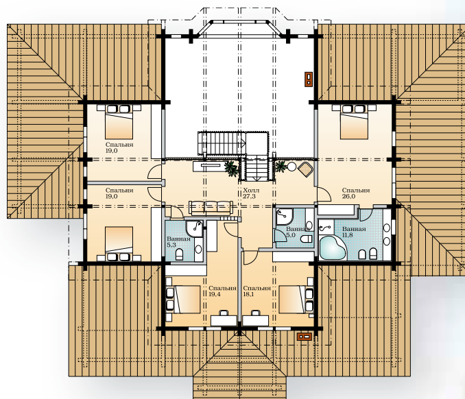
Второй этаж 1:300
