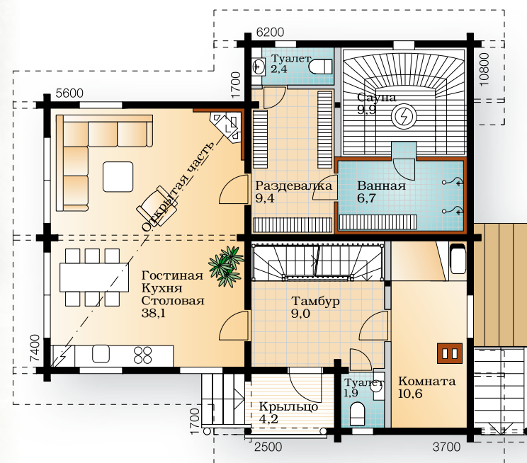
Первый этаж 1:150
