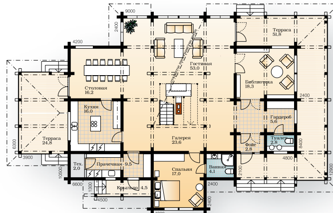
Первый этаж 1:300
