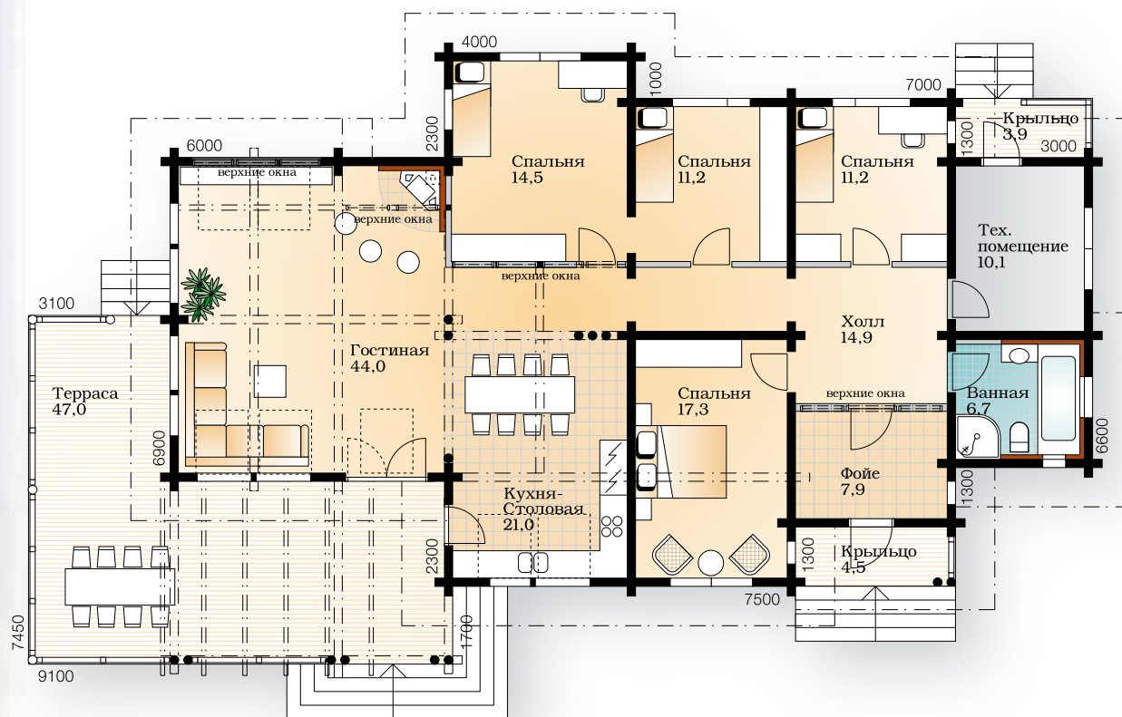
Первый этаж 1:150
