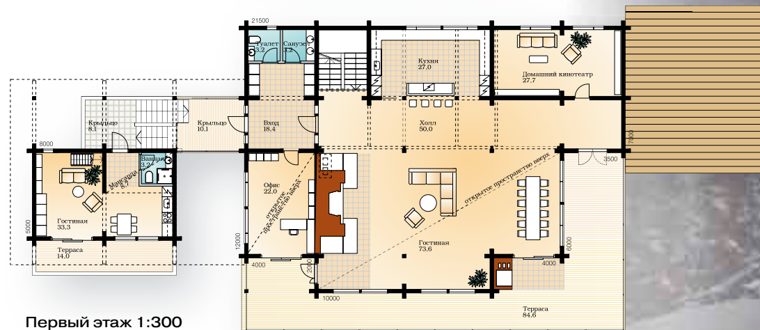
Первый этаж 1:300
