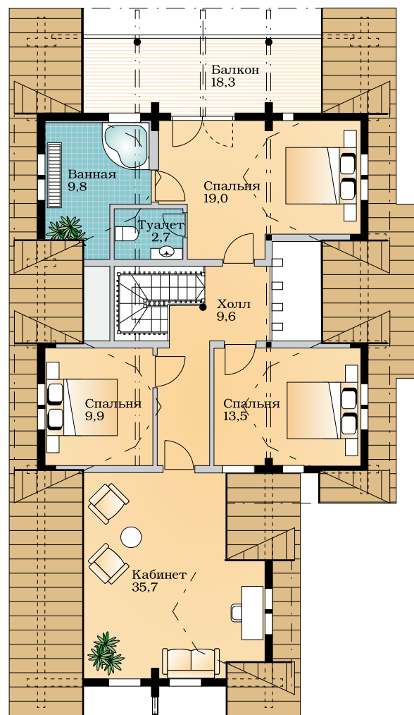
Второй этаж 1:150
