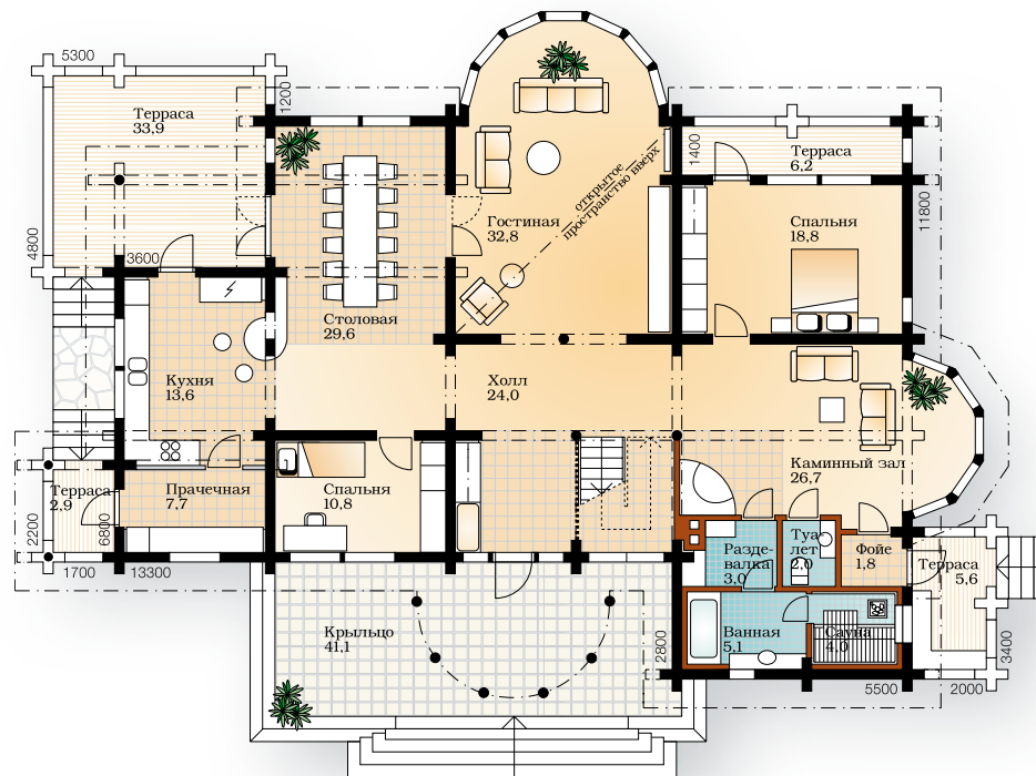
Первый этаж 1:200
