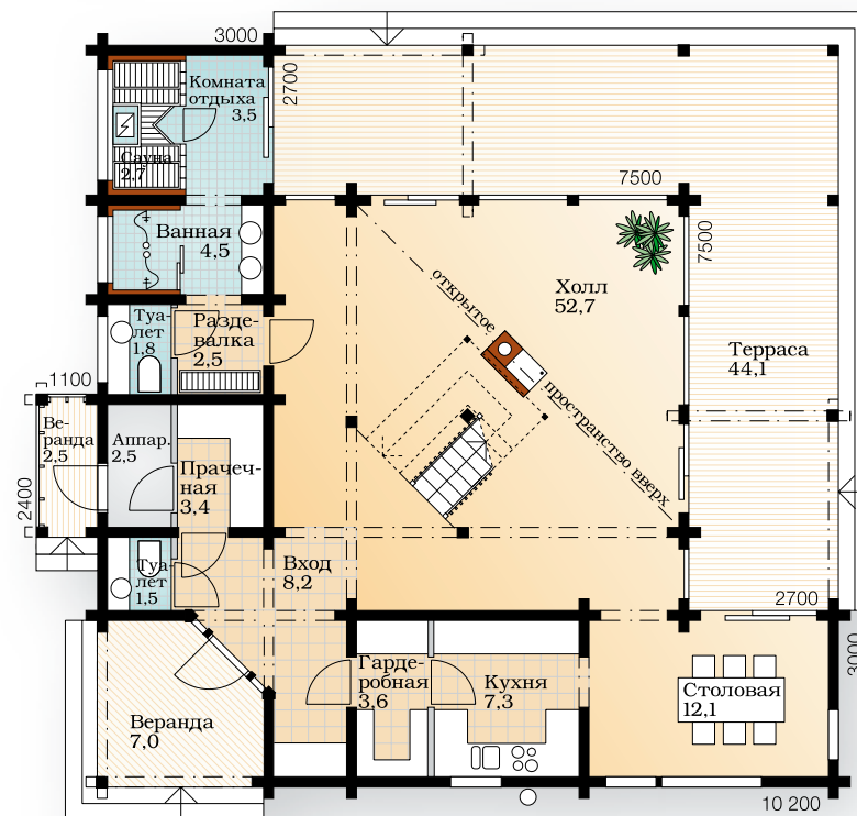
Первый этаж 1:150
