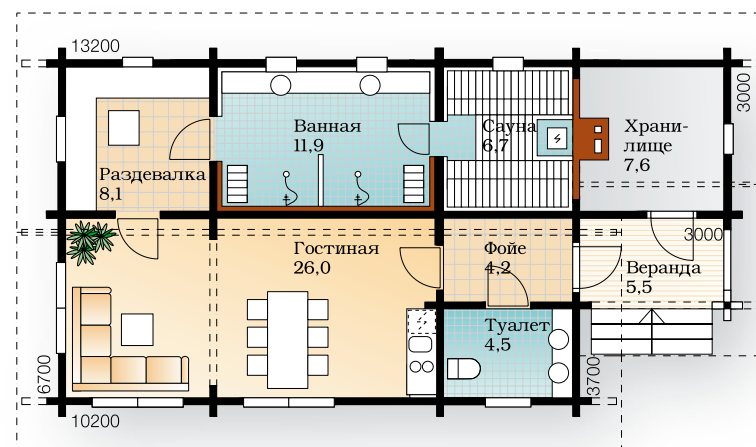
Первый этаж 1:150
