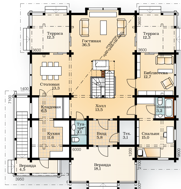
Первый этаж 1:200
