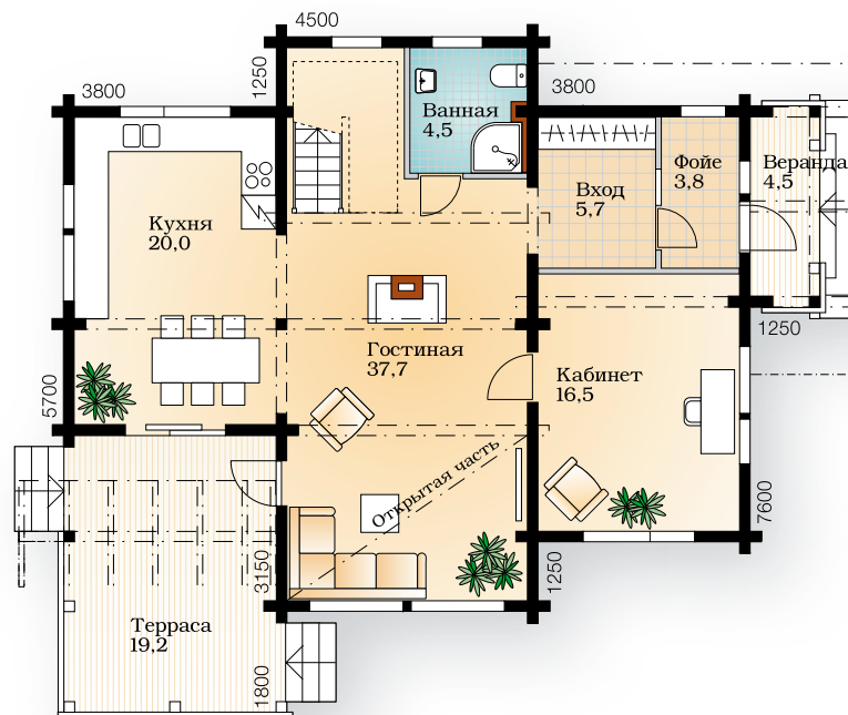
Первый этаж 1:150
