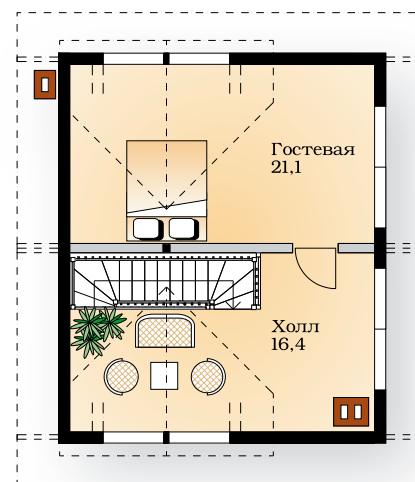
Второй этаж 1:150
