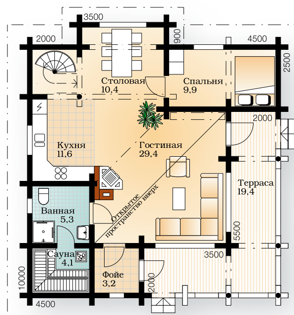
Первый этаж 1:150
