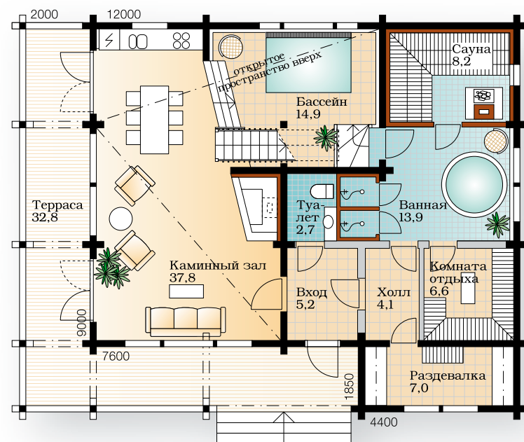
Первый этаж 1:150
