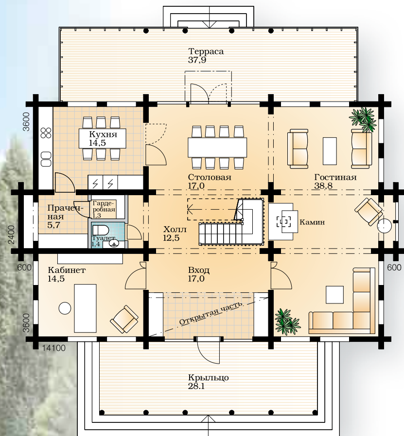
Первый этаж 1:150
