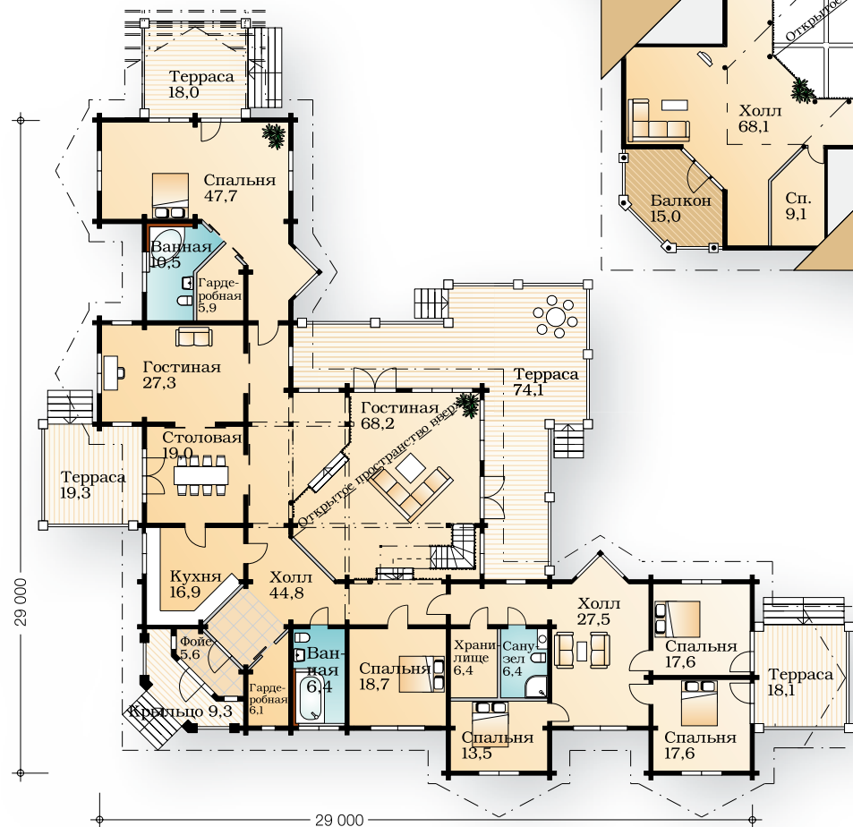
Первый этаж 1:300
