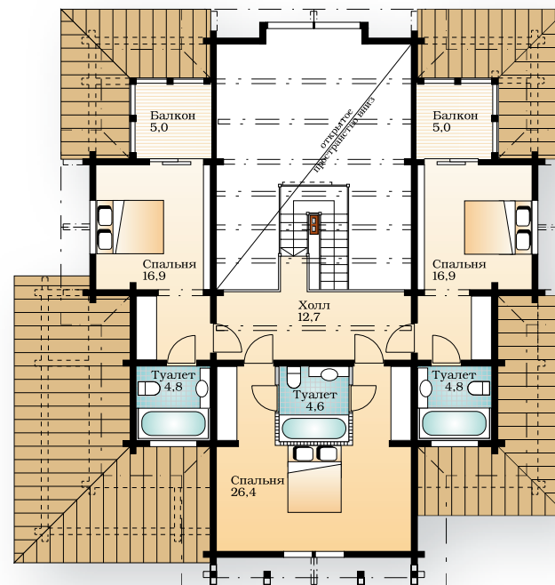
Второй этаж 1:200
