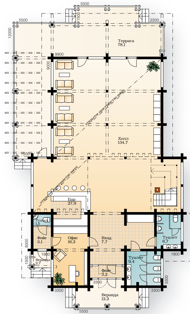
Первый этаж 1:200
