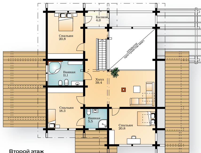
Второй этаж 1:200
