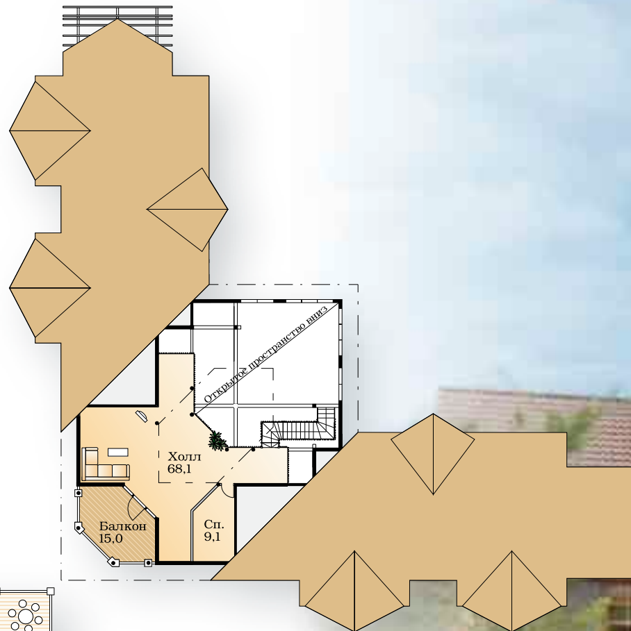
Второй этаж 1:300
