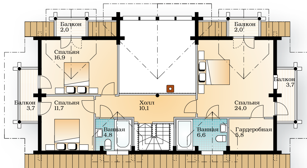
Второй этаж 1:150
