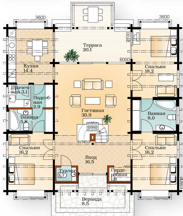
Первый этаж 1:150
